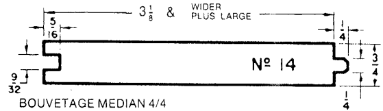
BOUVETAGE MEDIAN 4/4
