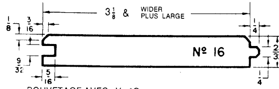
BOUVETAGE AVEC «V» 1C
