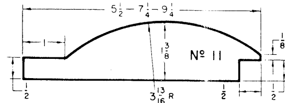
LAMBRIS DEMI-ROND 6/4
