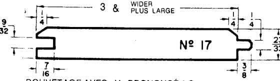
BOUVETAGE AVEC «V» PRONONCÉ 1C
