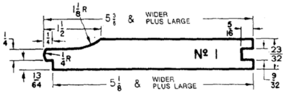
BOUVETAGE À GORGE
