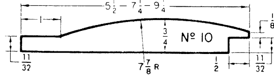
LAMBRIS DEMI-ROND 4/4
