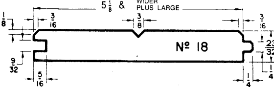
BOUVETAGE AVEC «V» MEDIAN 1C
