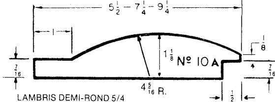
LAMBRIS DEMI-ROND 5/4
