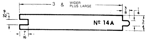
BOUVETAGE MEDIAN 4/4
