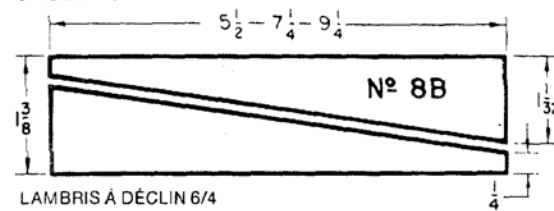
LAMBRIS À DÉCLIN 6/4
