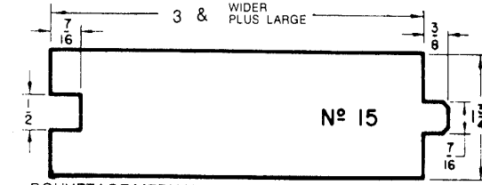
BOUVETAGE MEDIAN 8/4
