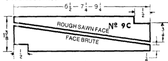
LAMBRIS À DÉCLIN 6/4; JOINT À MI-BOIS
