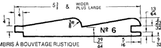
LAMBRIS À BOUVETAGE RUSTIQUE
