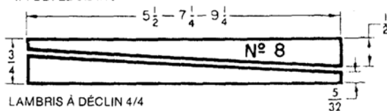
4/4 BEVEL SIDING
