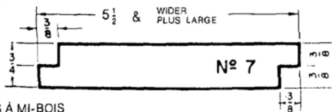
LAMBRIS À MI-BOIS
