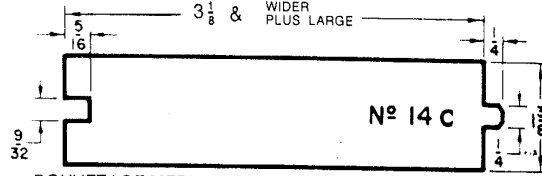
BOUVETAGE MEDIAN 6/4
